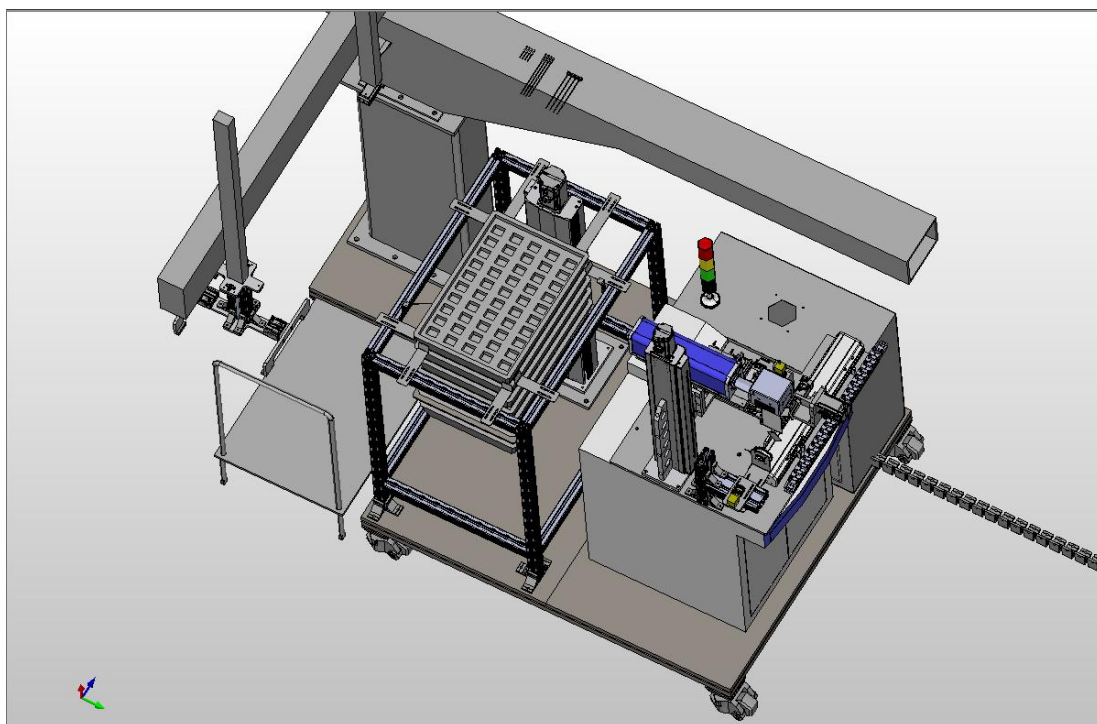
整机三维图
